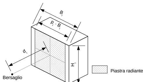
Illustrazione S.3-4: Schematizzazione della piastra radiante
